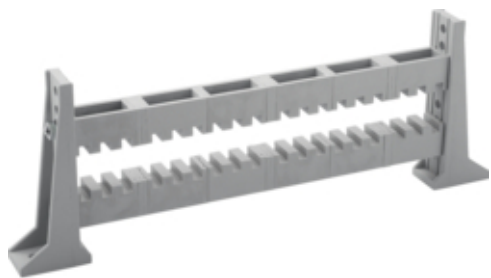
Schienenträger 4-polig Phasenmittenabstand 122.5mm
