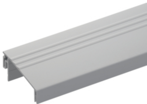
Wannenrandprofil zu R-T4 Länge 1.1m
