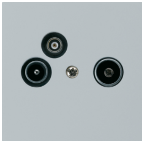
ka.A TV-données-radio 2GHz 4db
